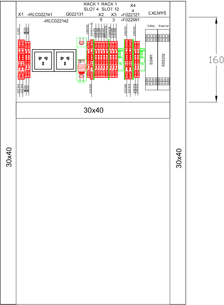
DETALLE A
